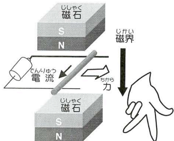
ず じかいちゆう お きんぞくぼう でんりゆう 図3 磁界中に置かれた金属棒に電流 たが きんぞくぼう みぎ へ を流すと金属棒が右に動く。
