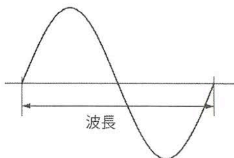
図5 光の波長
