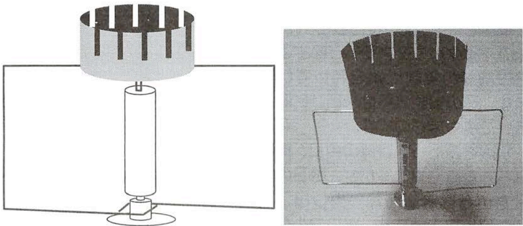
図15 クリップの上にゾートロープをセロハンテープで貼り付けます。
