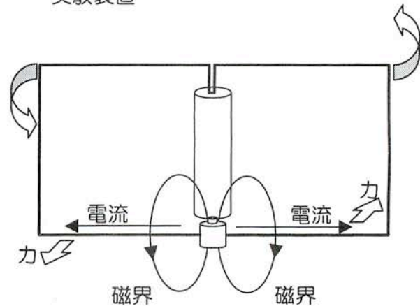
図16 たんきよく 単極モーターの原理 げんり
