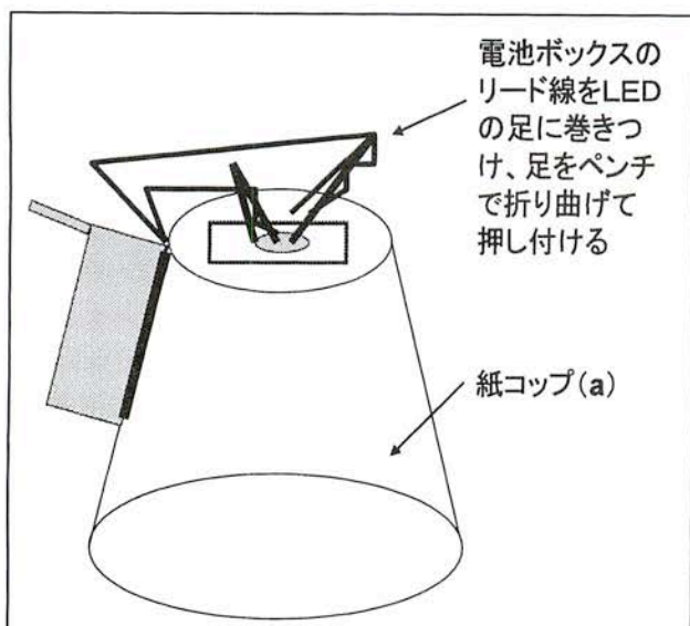
図8 電池ボックスからのリード線のLEDの足への配線。電池ボックスの赤い線をLEDの長い方の足に巻きつける。黒い線を短い方の足に巻きつける。その後、ラジオペンチでLEDの足を折り曲げて締め付けて、リード線がはずれないようにする。
