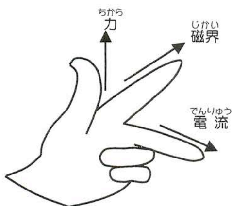
ず じかいちゆう なが でんりゆう はたら 図2 磁界中を流れる電流に働く ちから ひだりて ほうそく 力 (フレミングの左手の法則)
